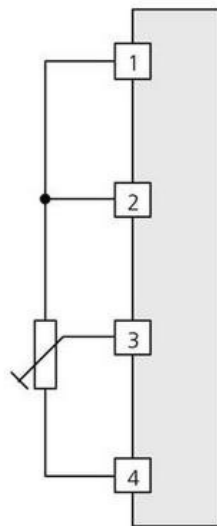
4 vodičový obvod
