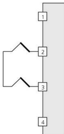
Termočlánky pro diferenční měření
