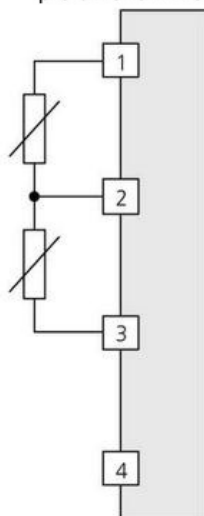
RTD 3 vodičové připojení pro diferenční měření
