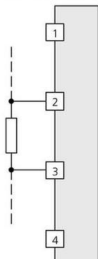
Měření proudu s bočníkem
