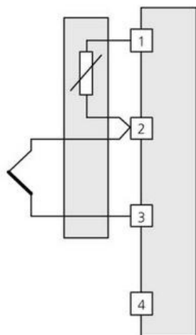
Termočlánek s externí kompenzací studeného konce
