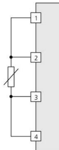
RTD 4 vodičové připojení
