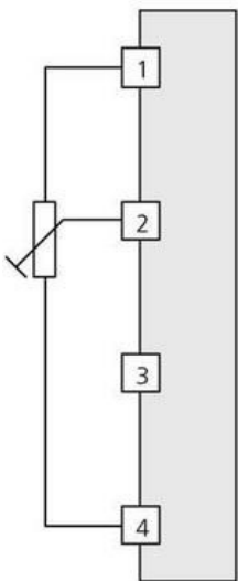
3 vodičový obvod
